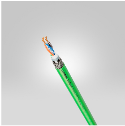
LAPP KABEL STUFGART ETHERLINE® PN Cat.6. FLEX FC 4x2xAWG23/7
